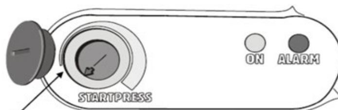
НАСТРОЙКА ДАВЛЕНИЯ ВКЛЮЧЕНИЯ
